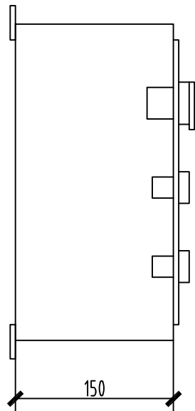
侧视图
