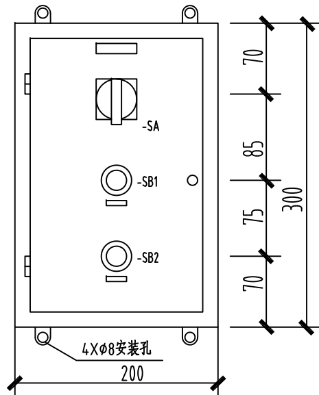
正视图
