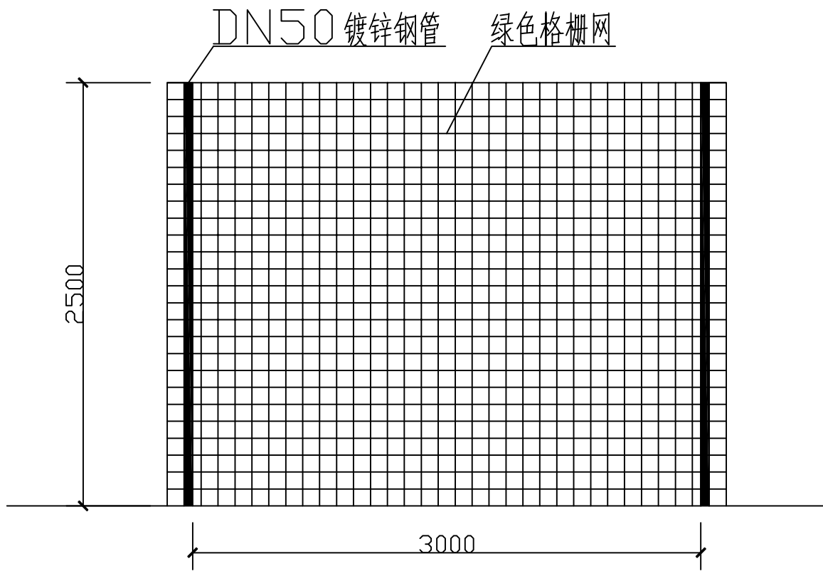
防护栏正面示意图
