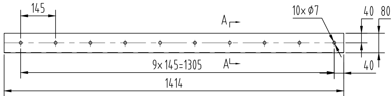
U型绝缘槽板(材料为SMC)
