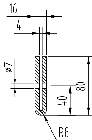
U型绝缘槽板截面
