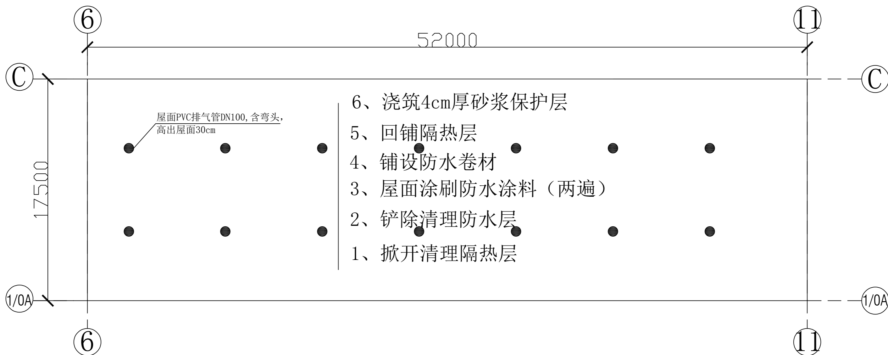
屋面做法示意图
